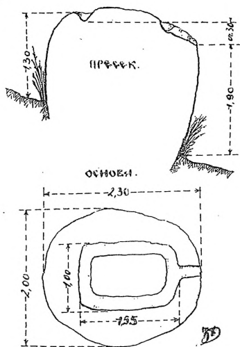
Сл. 2. — Основа и пресек гранитног жртвеника.
