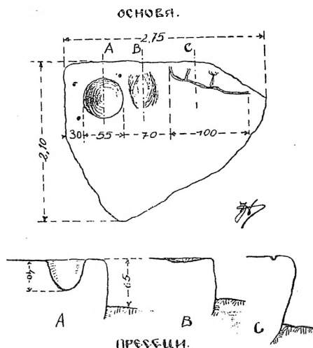
Сл. 4. — Основа и пресеци гранитног мегалита.
